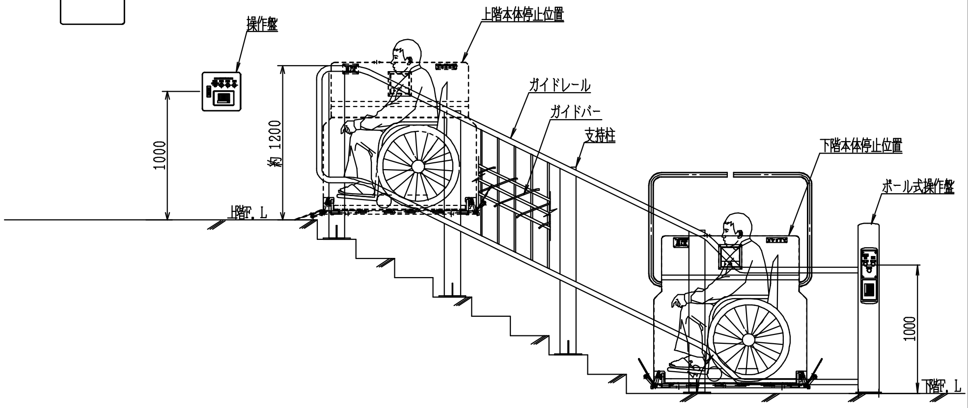
階段 断面図
