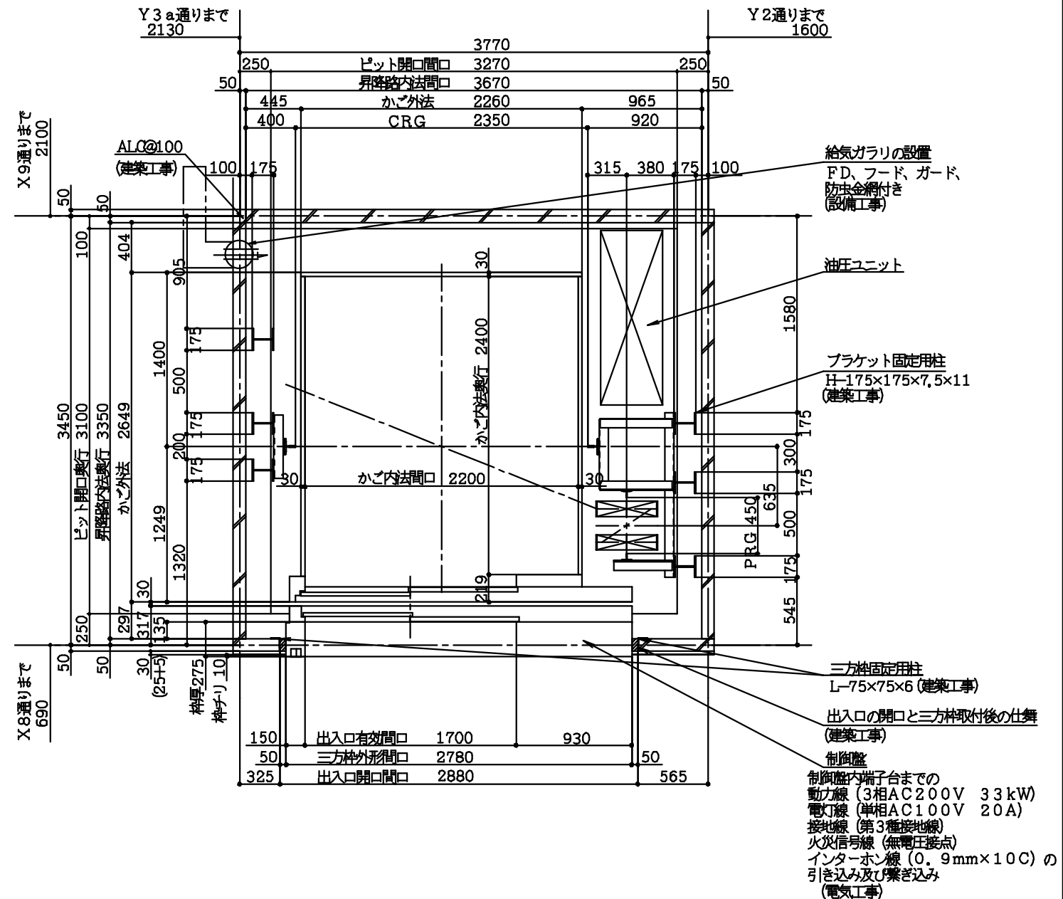
1階昇降路平面図 S=1/30
